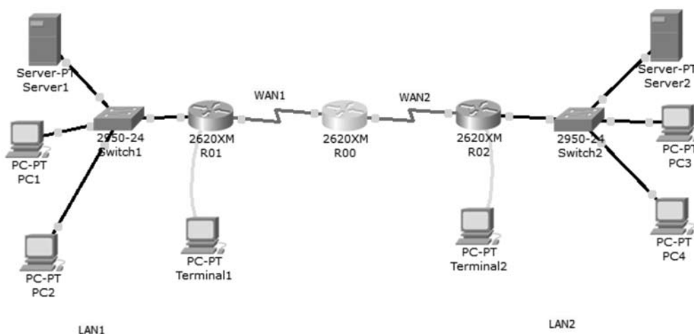
Rysunek 51. Schemat topologii sieci dla routingu statycznego
