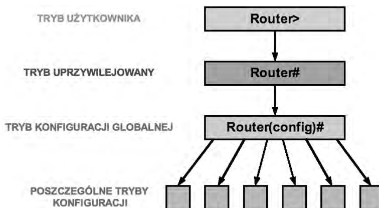
Rysunek 12. Tryby konfiguracji routera
