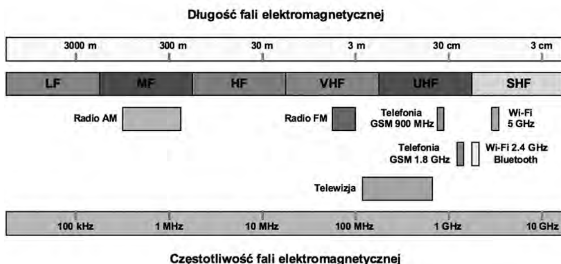
Rysunek 1. Spektrum fal elektromagnetycznych
