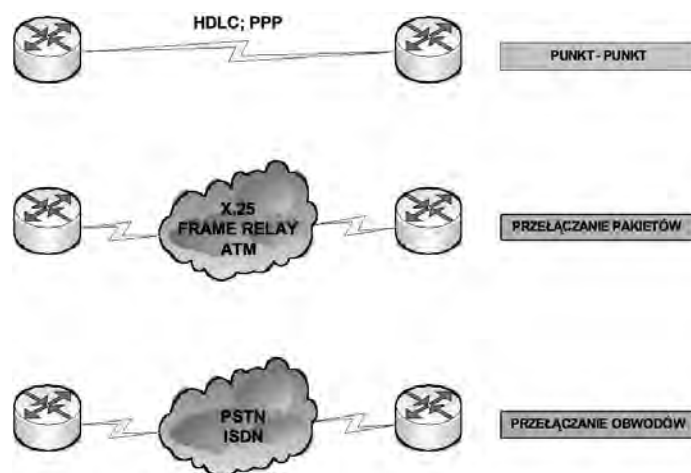
Rysunek 5. Przykłady połączeń w sieciach WAN
