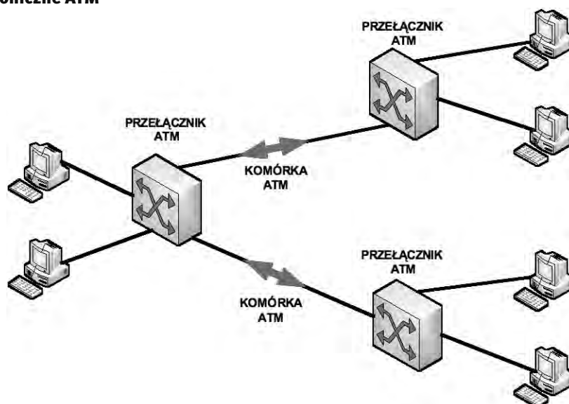
Rysunek 14. Przełączanie komórek w sieciach ATM
